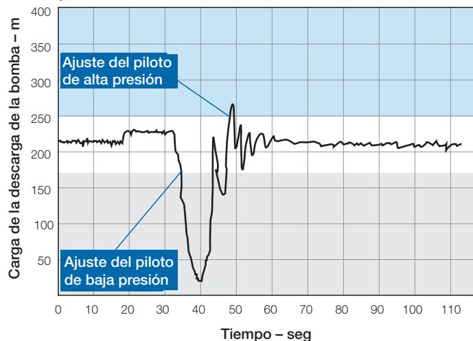
Presión en la estación de bombeo protegida por la válvula Modelo 735-M
